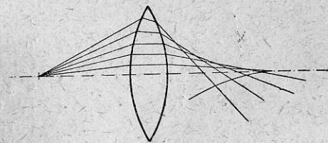
Рис. 11. Сферическая аберрация. Лучи, выходящие из одной точки, не пересекаются в одной точке. Различные точки пересечения лучей лежат на разных расстояниях от центра линзы.
