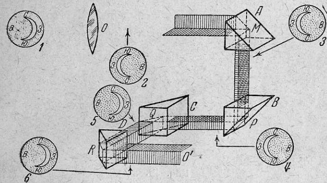
Рис. 18. Схема призменного бинокля;
