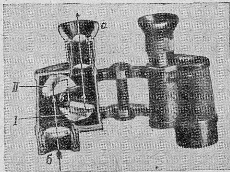
Рис. 17. Ход лучей в призменном бинокле: a — окуляр; b — объектив; e — призмы.
